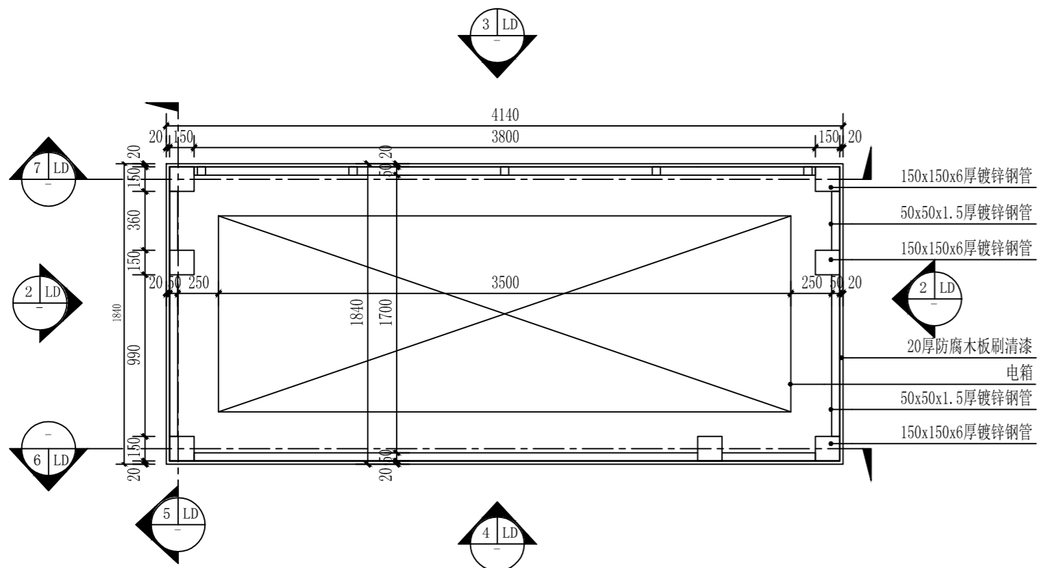
1 电箱平面图 1:30
