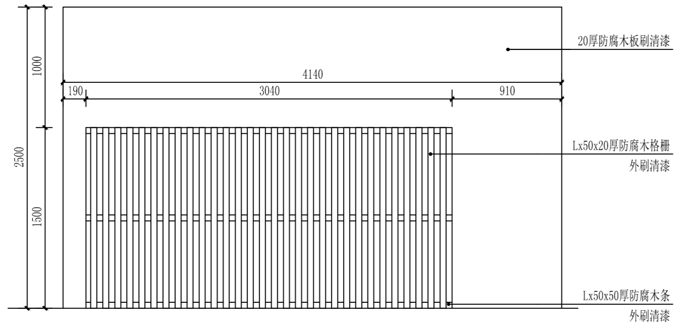
4 立面图三 1:30
