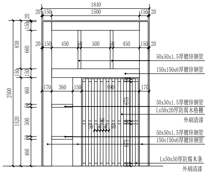
2 立面图一 1:30
