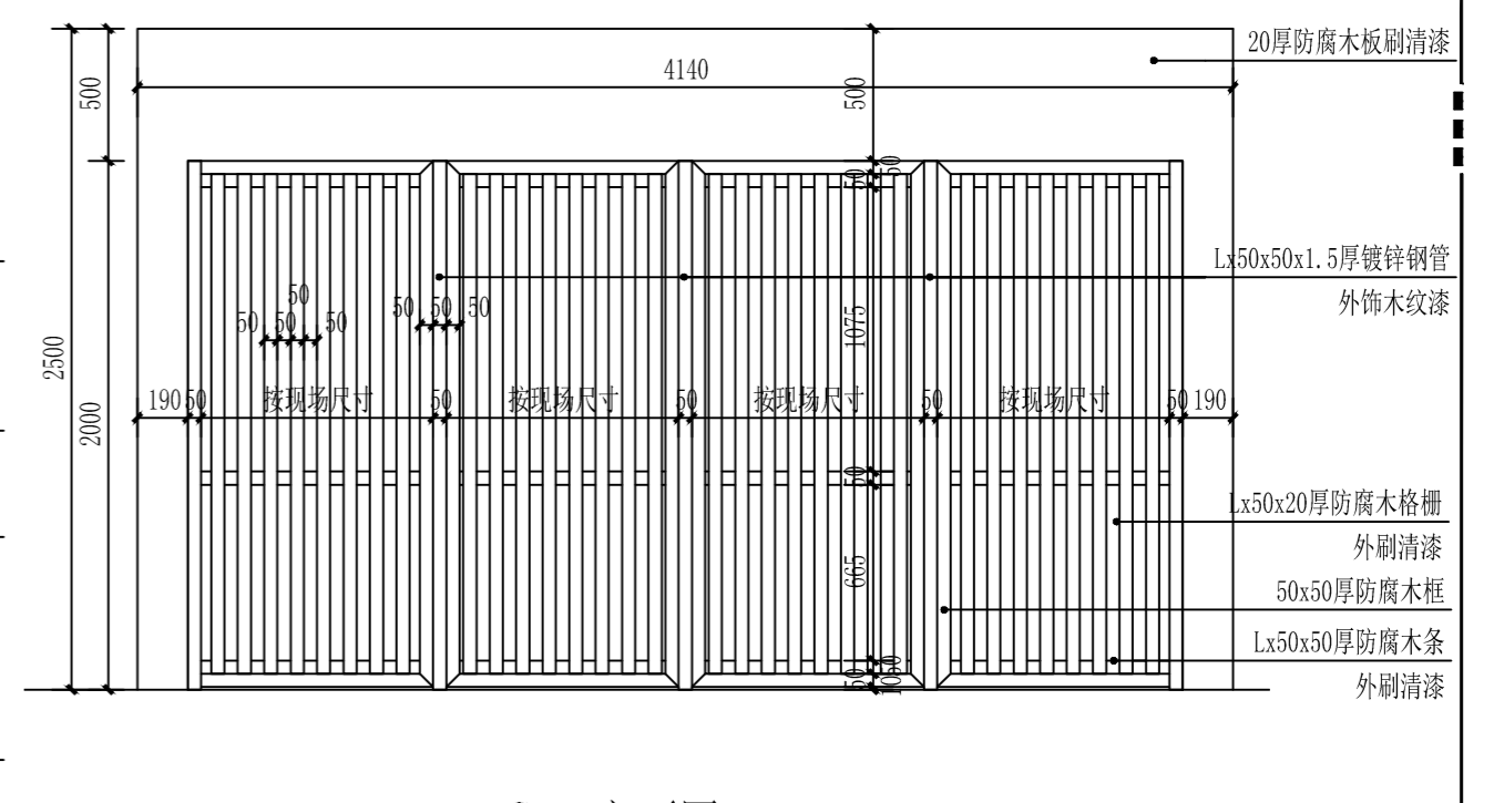
3 立面图二 1:30
