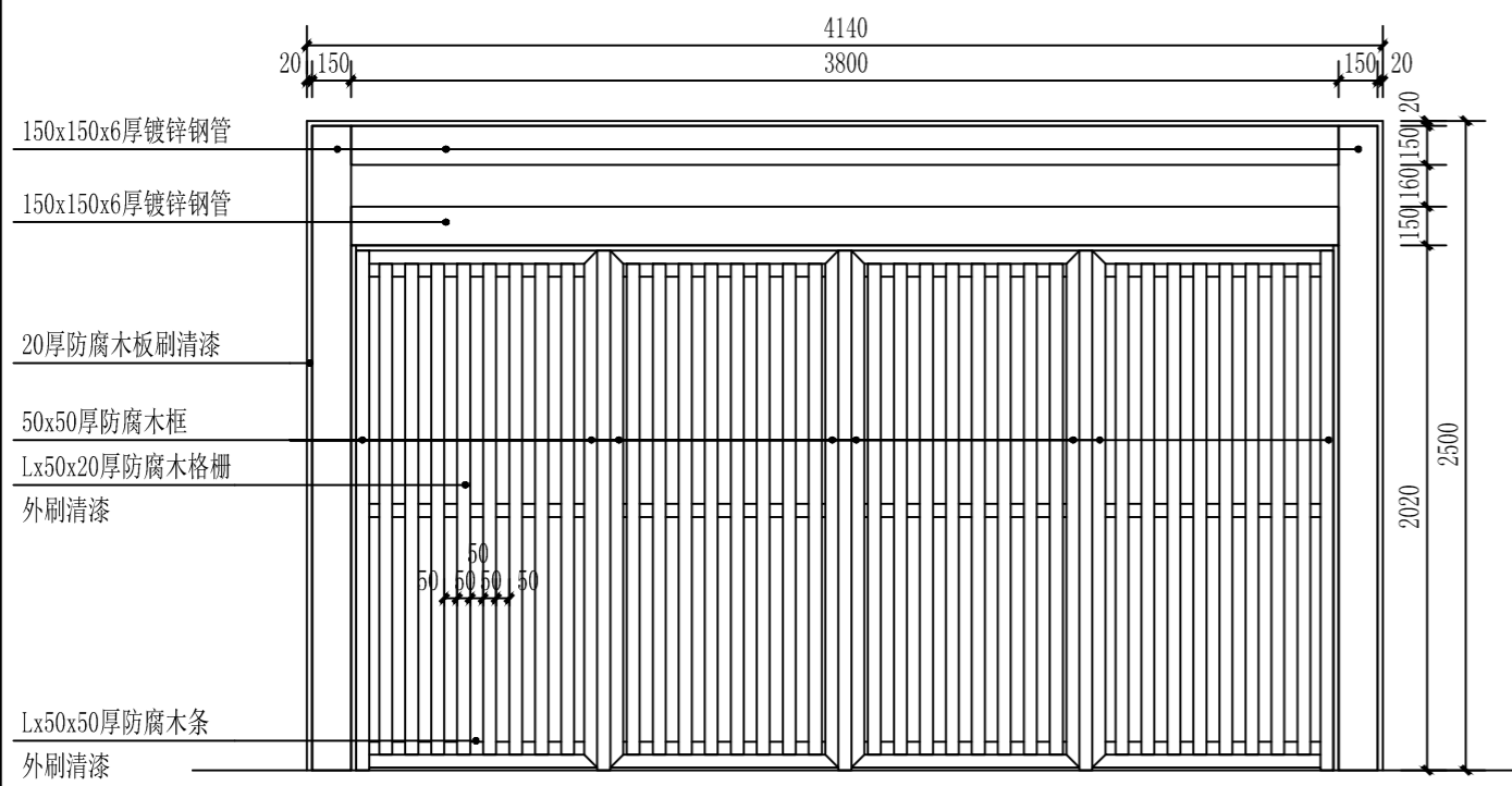
7 做法三 1:30
