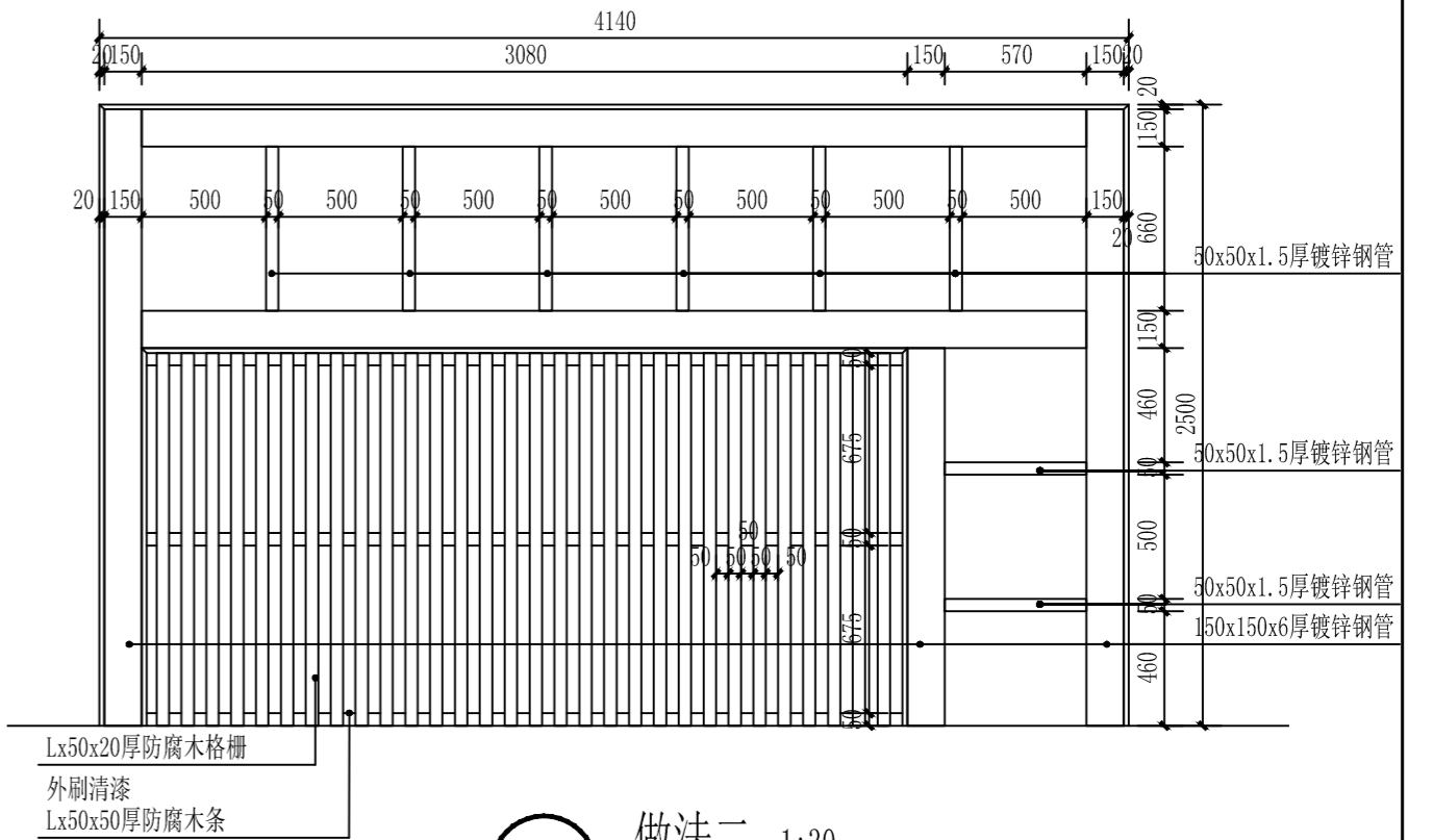
6 做法二 1:30
