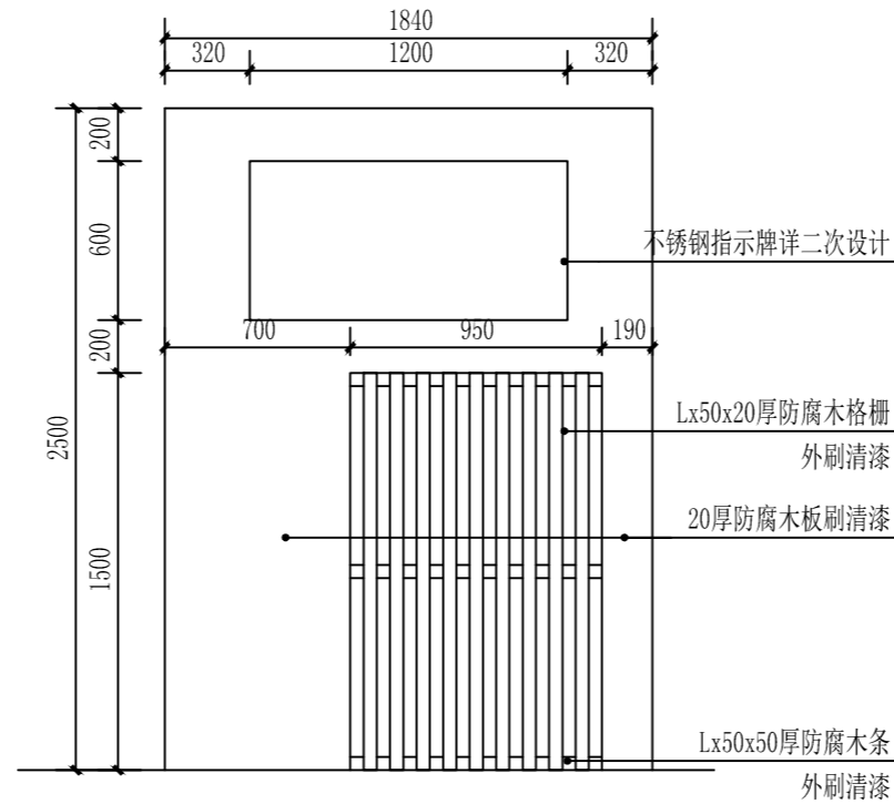
2 立面图一 1:30
