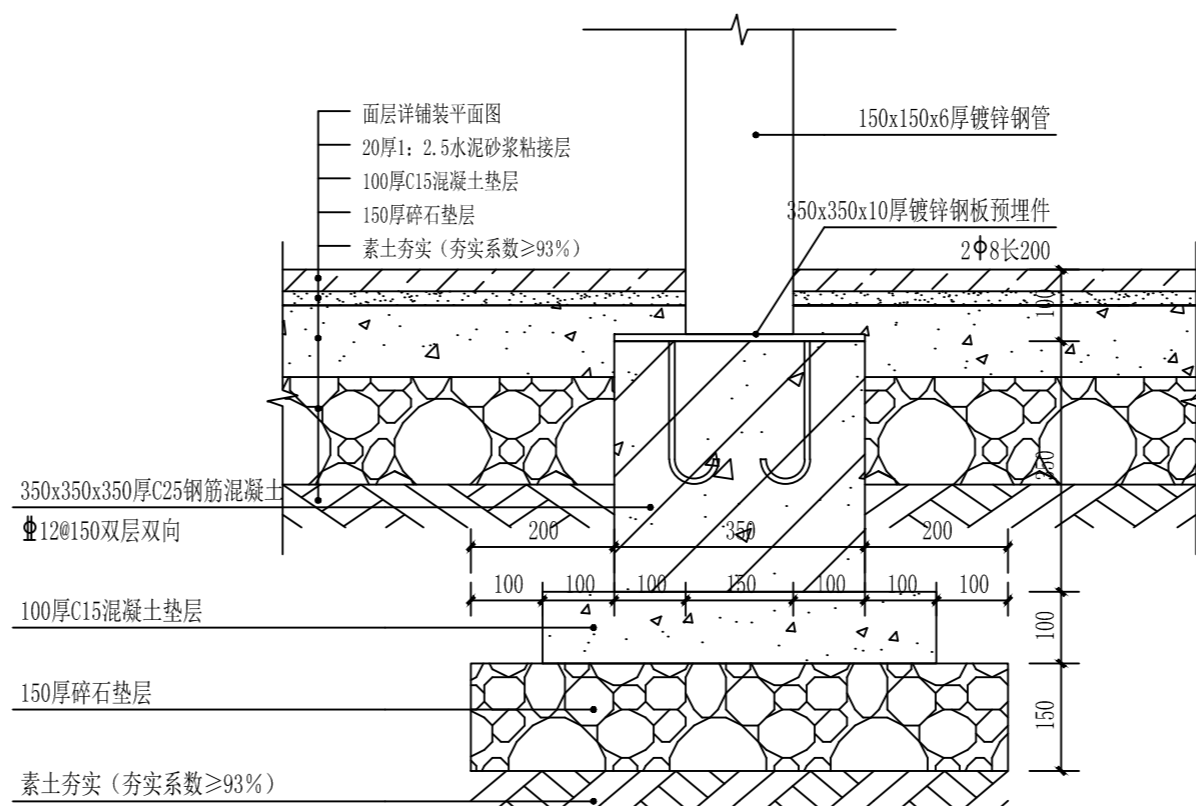
8 基础做法图 1:10
